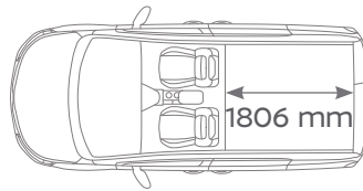
Rakodási hossz
