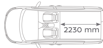
Rakodási hossz
